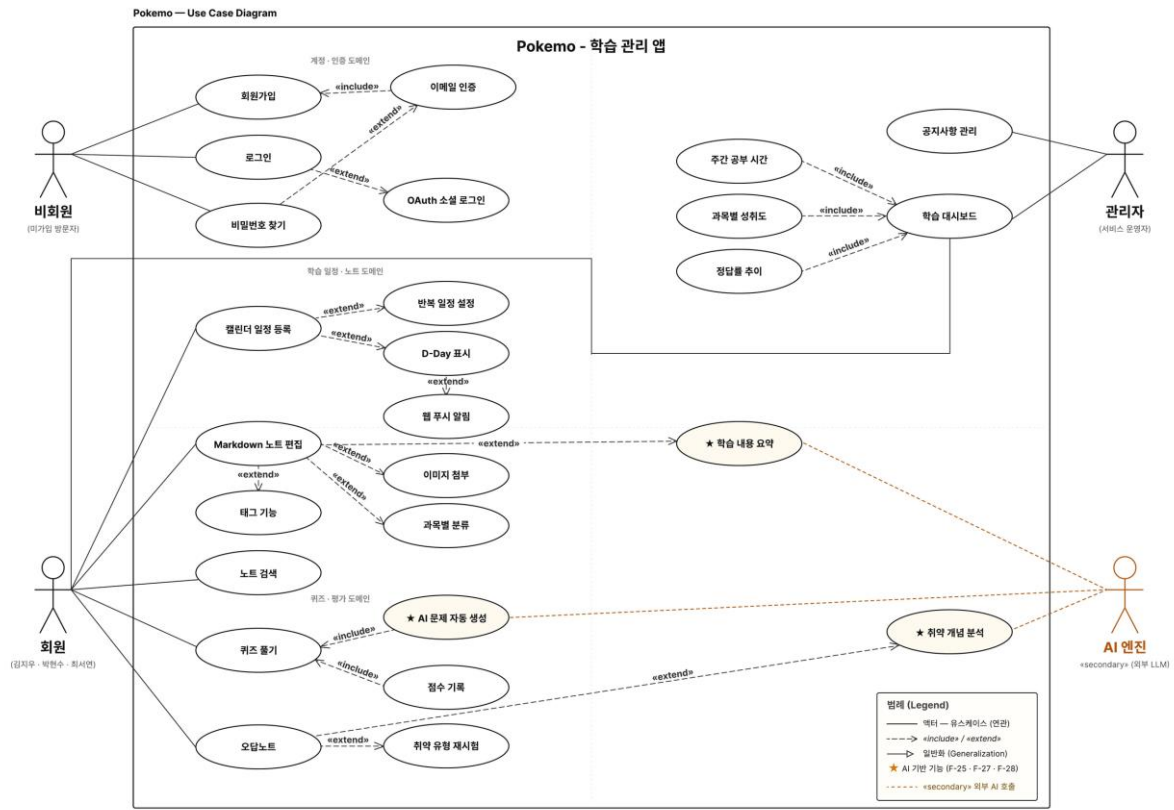
[그림 4-1] Pokemo 유스케이스 다이어그램
