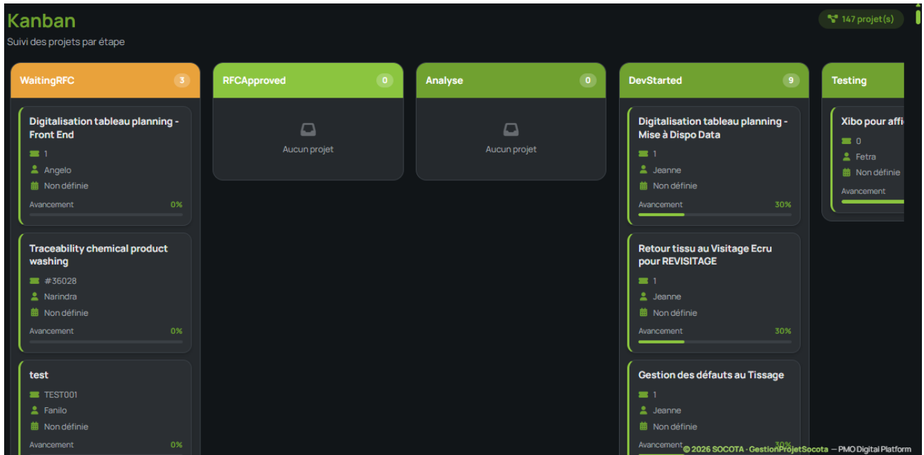
Figure 5 — Vue Kanban.
