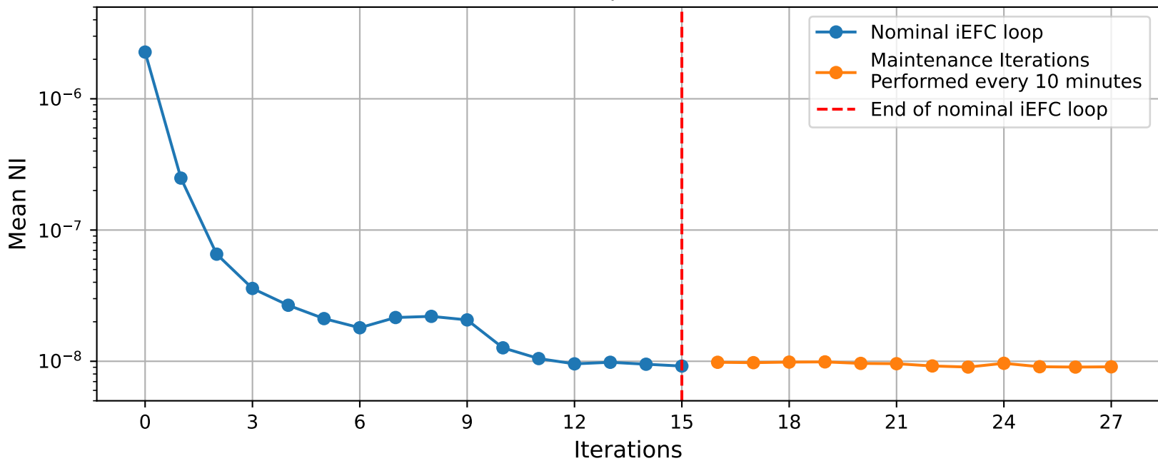
Contrast per Iteration
