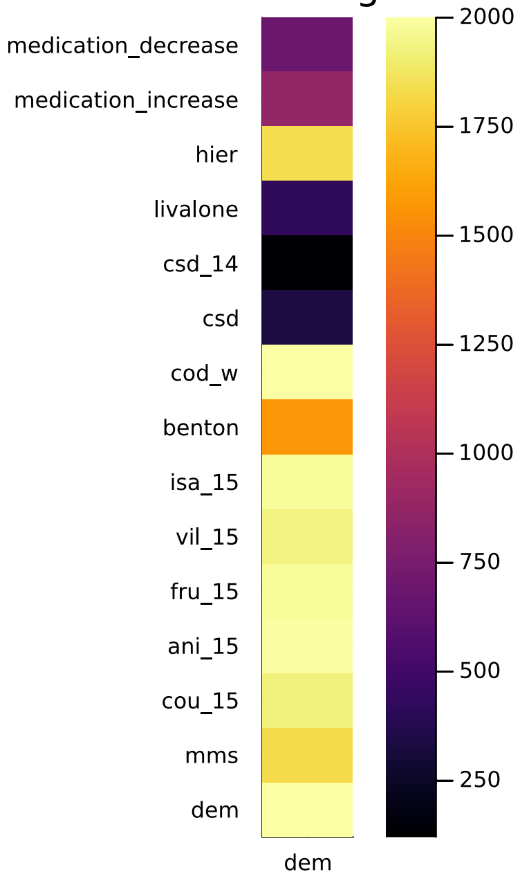
dem: lag0
