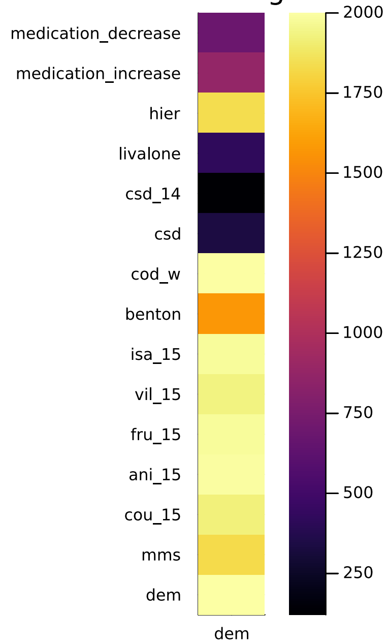
dem: lag2
