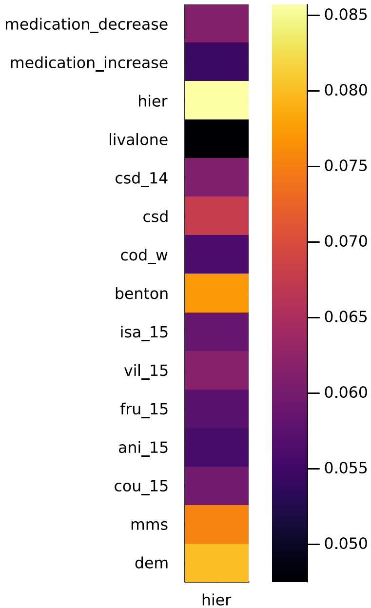
hier: lag1
