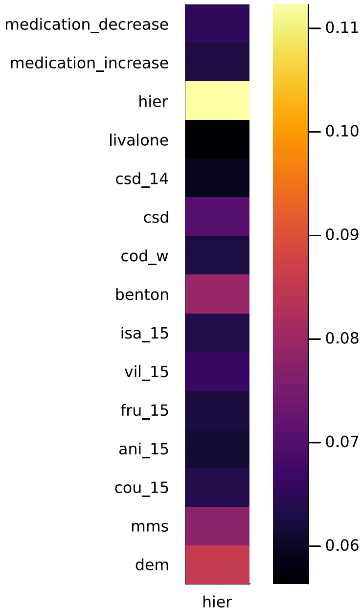
hier: lag0
