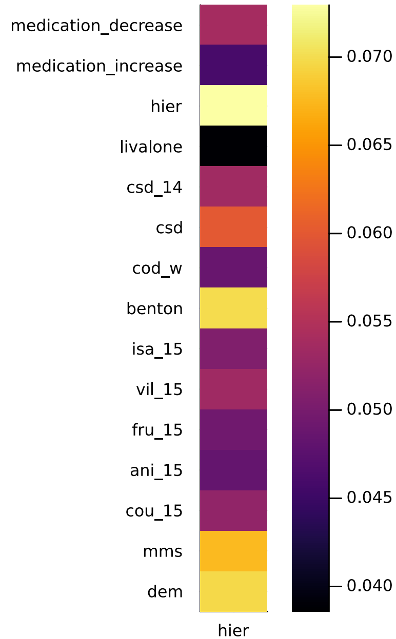
hier: lag2
