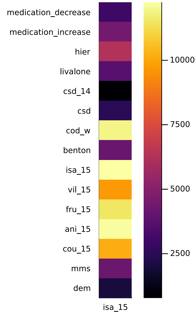
isa_15: lag2
