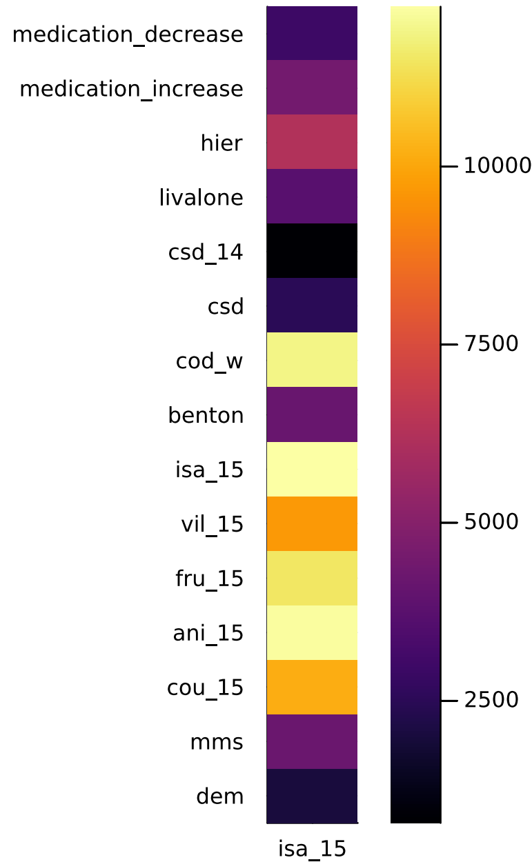
isa_15: lag1
