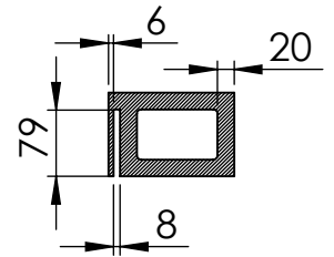
SECCIÓN A-A ESCALA 1 : 10
