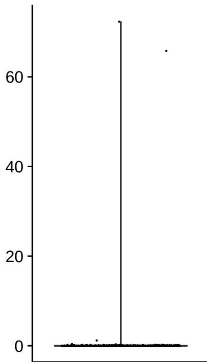
percent.hb
