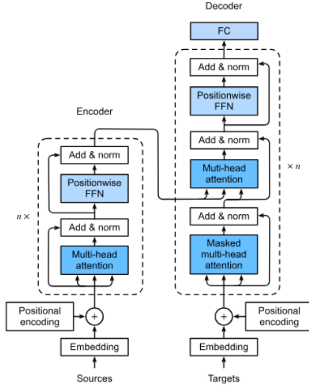
Hình 2.3: Kiến trúc Transformer [34] với hai thành phần chính: bộ mã hóa (trái) xử lý chuỗi nguồn qua n lớp gồm cơ chế chú ý đa đầu và mạng truyền thẳng theo vị trí với kết nối tắt; bộ giải mã (phải) tổng hợp đặc trưng từ bộ mã hóa để sinh chuỗi đích thông qua cơ chế chú ý đa đầu có mặt nạ và cơ chế chú ý chéo.
