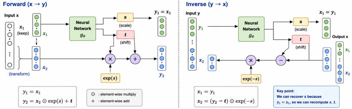
Hình 2.5: Cấu trúc một khối INN (Affine Coupling Layer): chiều thuận (trái sang phải) và chiều nghịch (phải sang trái) đều tính được hiệu quả. (Nguồn: [19])
