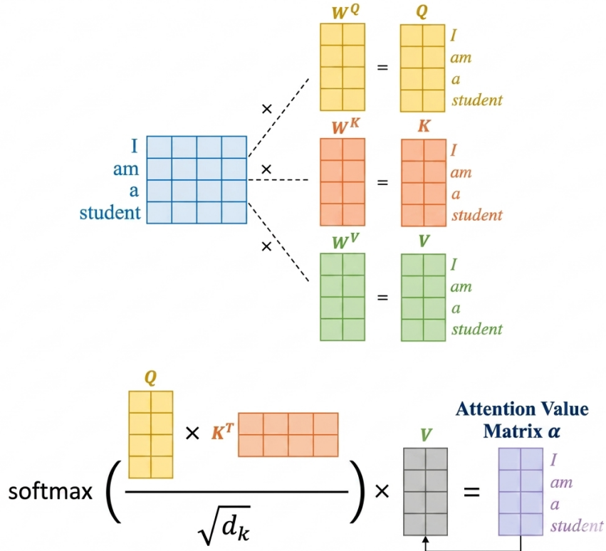
Hình 2.3: Sơ đồ Scaled Dot-Product Attention: Q , K , V qua các bước nhân ma trận, chia tỉ lệ và softmax để tạo ra đặc trưng đầu ra. (Nguồn: [16])
