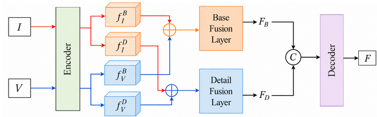
Hình 2.6: Kiến trúc tổng quan CDDFuse: hai ảnh đầu vào đi qua Encoder dùng chung trọng số, phân rã thành đặc trưng Base ( f^B ) và Detail ( f^D ), được tổng hợp riêng qua Fusion Layer, rồi giải mã thành ảnh đầu ra I_F . (Nguồn: [1])
