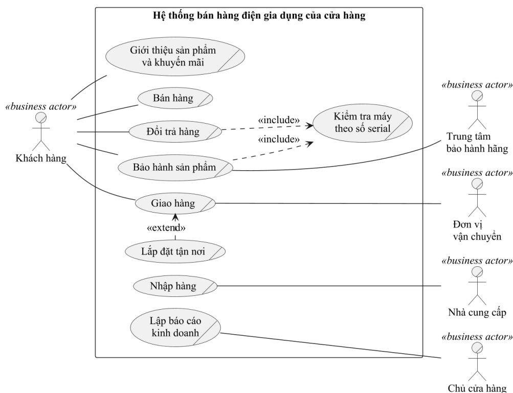
Hình 3.2: Sơ đồ use case nghiệp vụ tổng (bản nháp)
