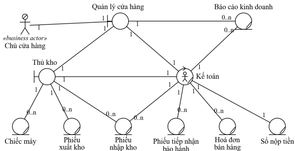
Hình 3.9: Sơ đồ đối tượng nghiệp vụ BUC-07 Lập báo cáo kinh doanh
