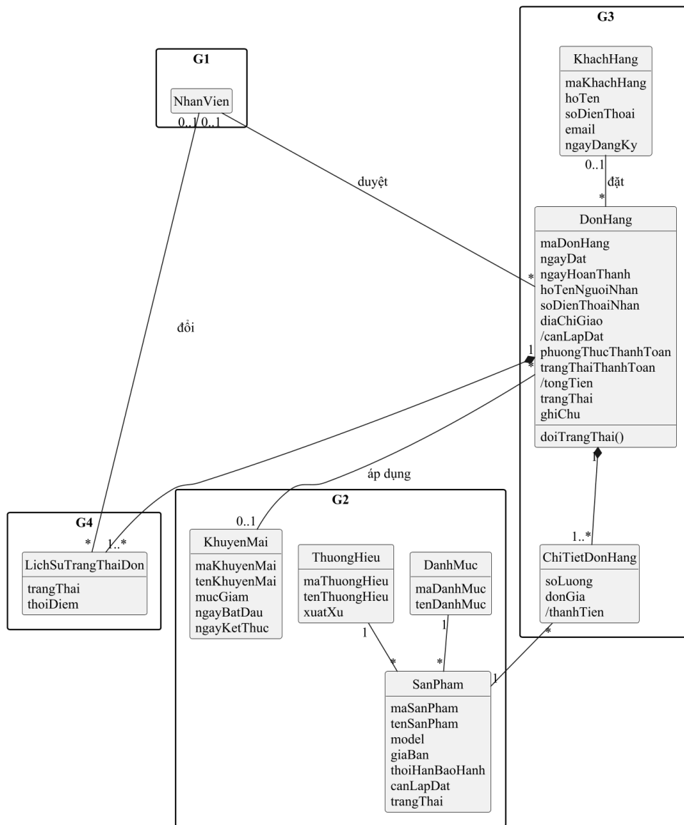
Hình 3.7: Lớp dùng chung, phần bán hàng (bản nháp)
