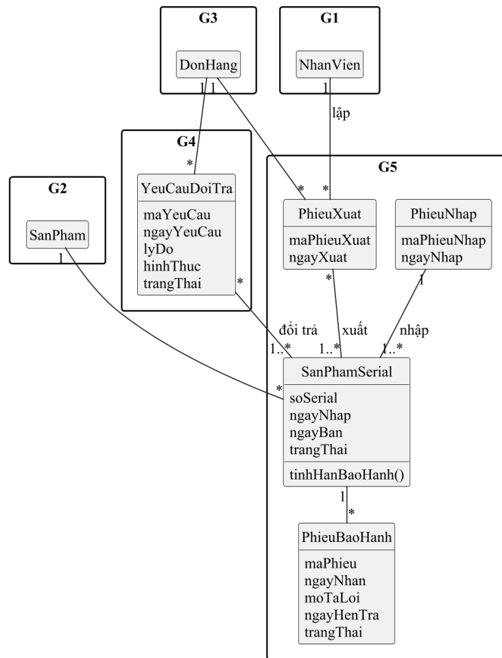
Hình 3.8: Lớp dùng chung, phần theo dõi chiếc máy (bản nháp)
