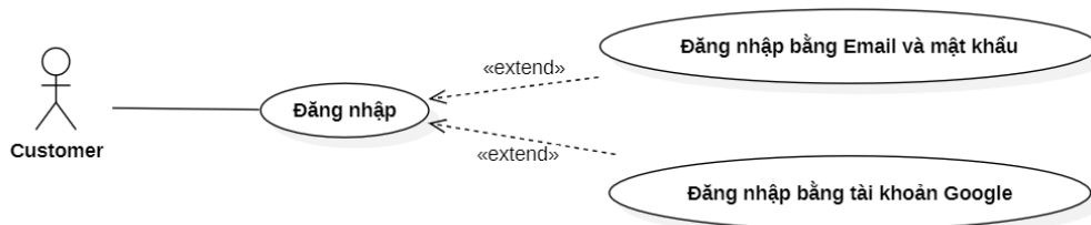
Hình 3.5 Sơ đồ use-case đăng nhập
