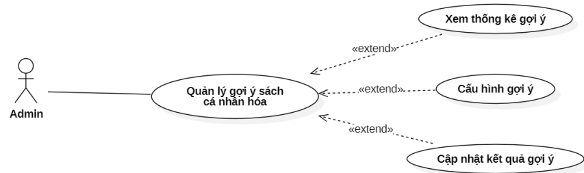
Hình 3.15 Sơ đồ use-case quản lý gợi ý sách cá nhân hóa
