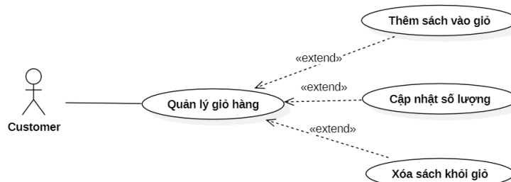
Hình 3.9 Sơ đồ use-case quản lý giỏ hàng
