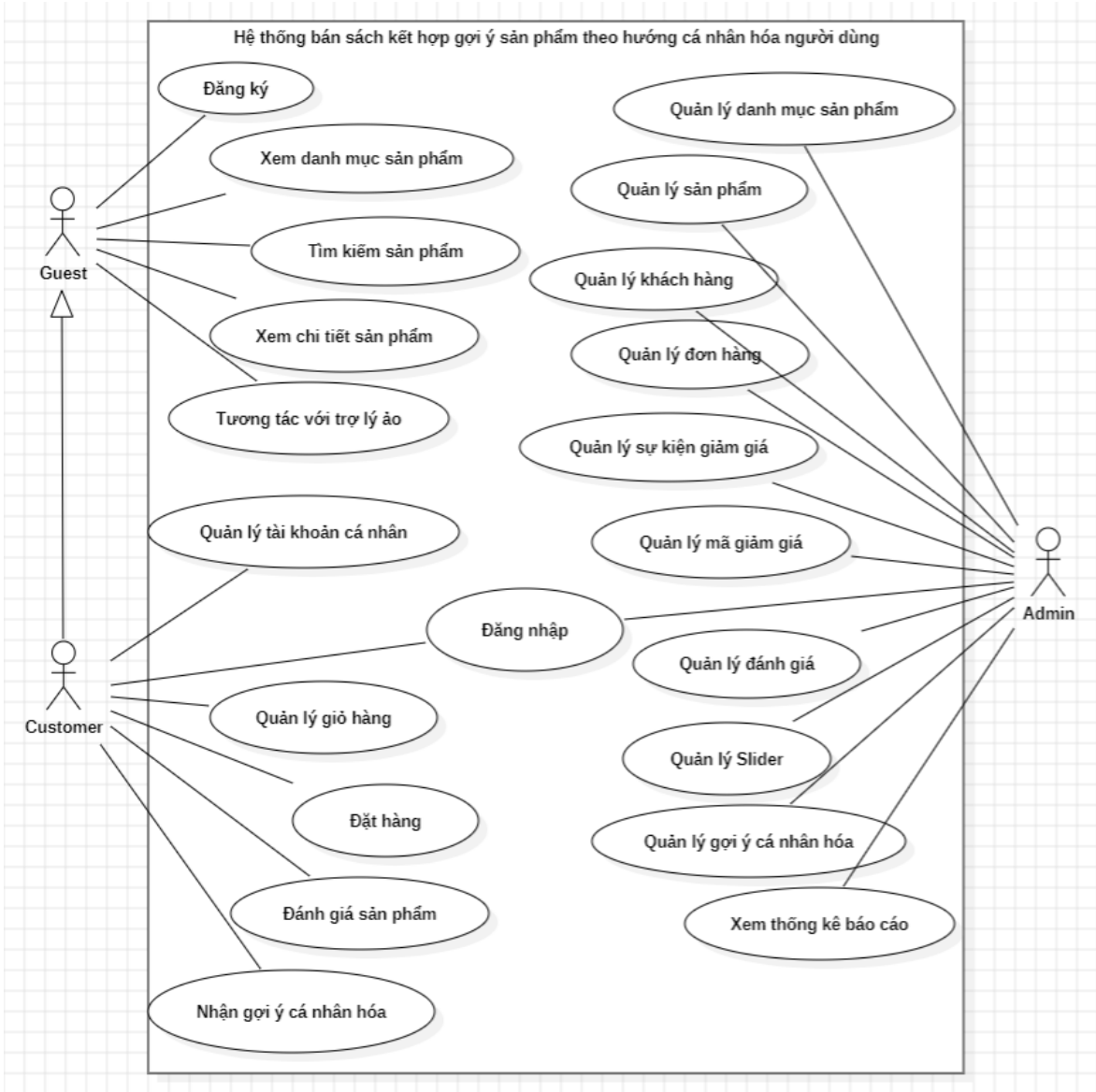
Hình 3.3 Sơ đồ use-case tổng quát
