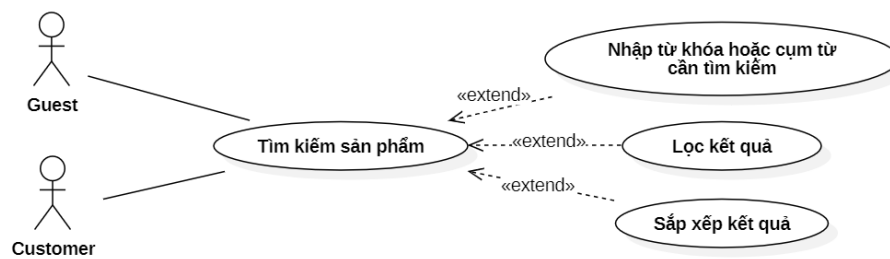
Hình 3.6 Sơ đồ use-case tìm kiếm sản phẩm
