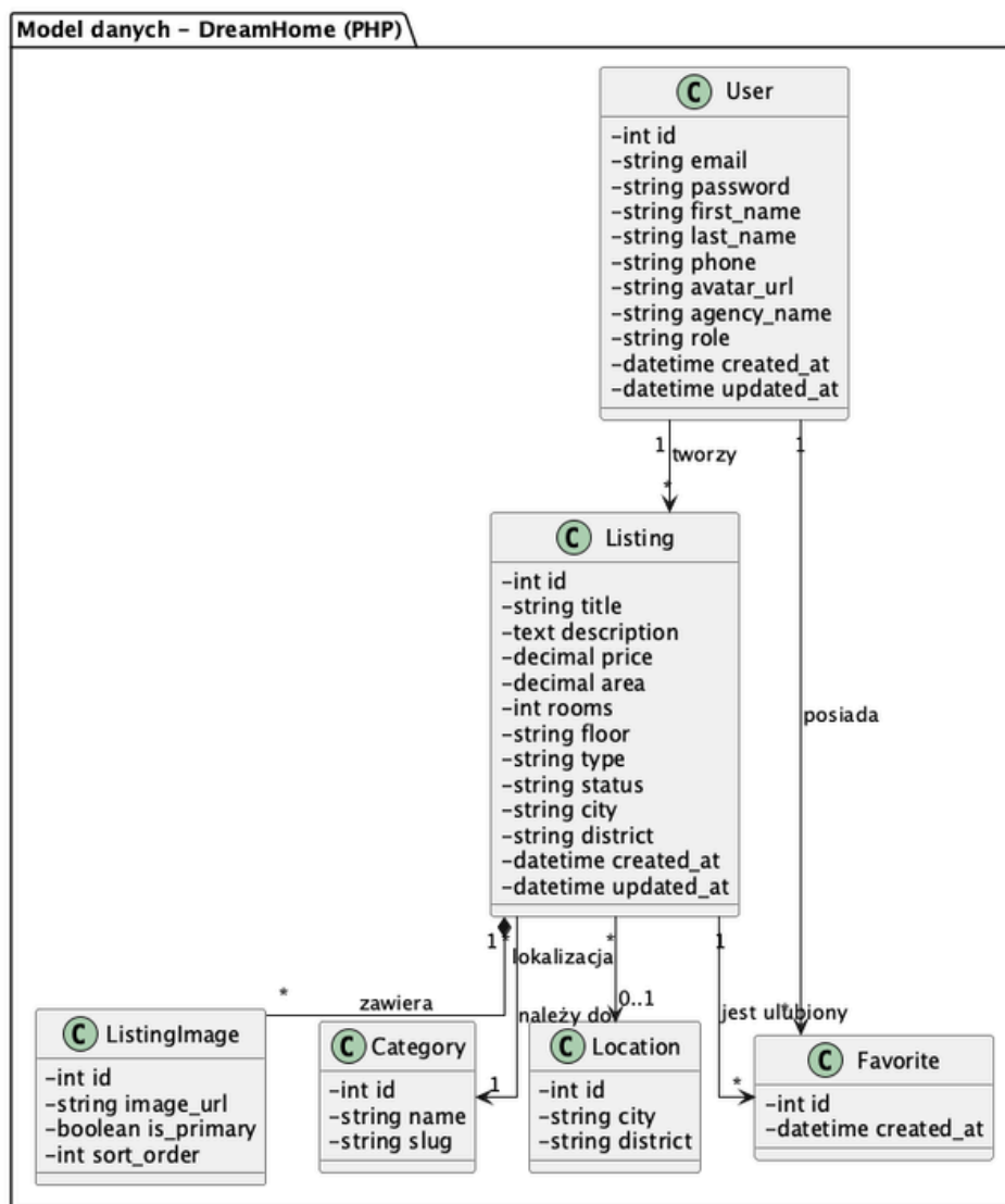
Rysunek 2: Diagram klas - modele Eloquent
