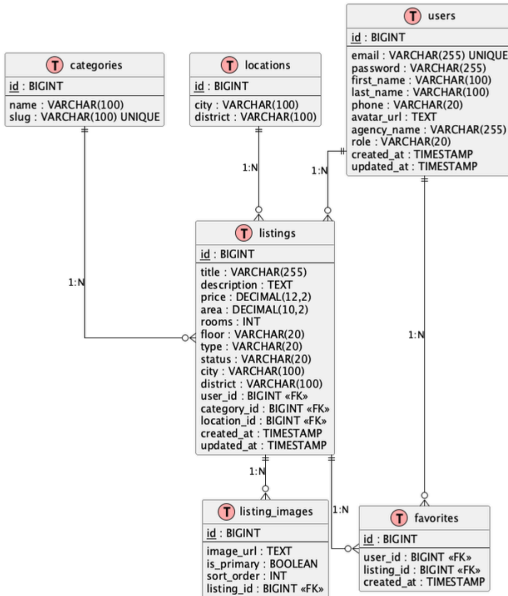
Rysunek 3: Diagram relacji encji (baza danych)
