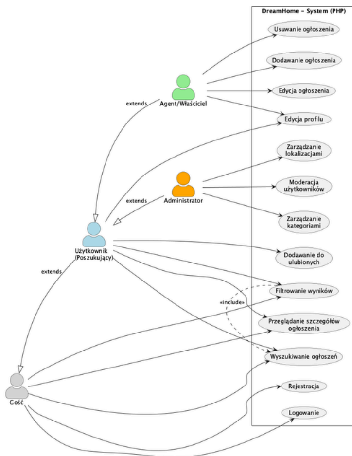
Rysunek 1: Diagram przypadków użycia - DreamHome PHP
