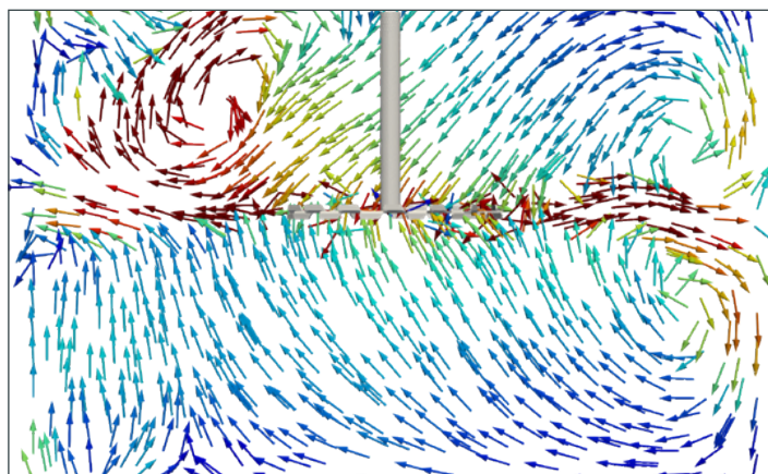
LÍNEAS DE FLUJO | REPRESENTACIÓN DISCO COWLES
