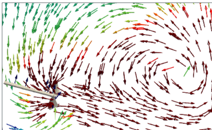
LÍNEAS DE FLUJO | REPRESENTACIÓN HÉLICE SABRE
