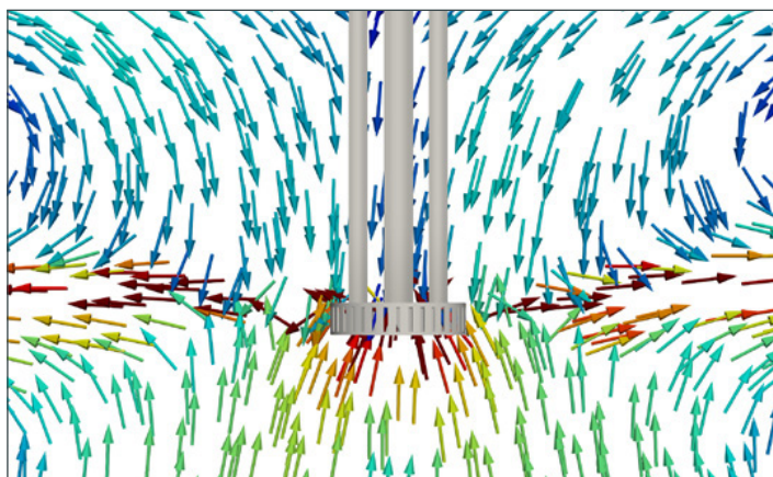
LÍNEAS DE FLUJO | REPRESENTACIÓN ROTOR-ESTATOR
