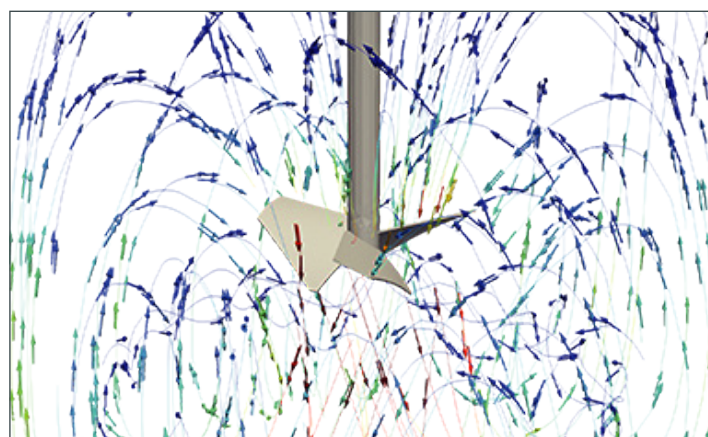
LÍNEAS DE FLUJO | REPRESENTACIÓN HÉLICE NABLA
