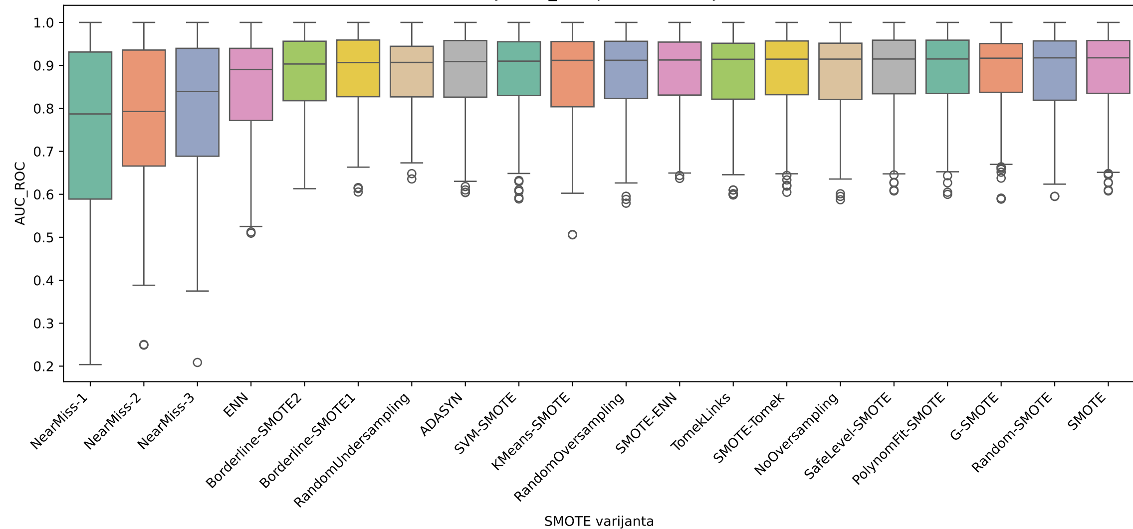
Distribucija AUC_ROC po SMOTE varijantama
