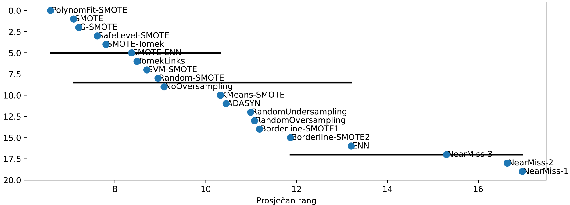
CD dijagram — AUC_ROC
