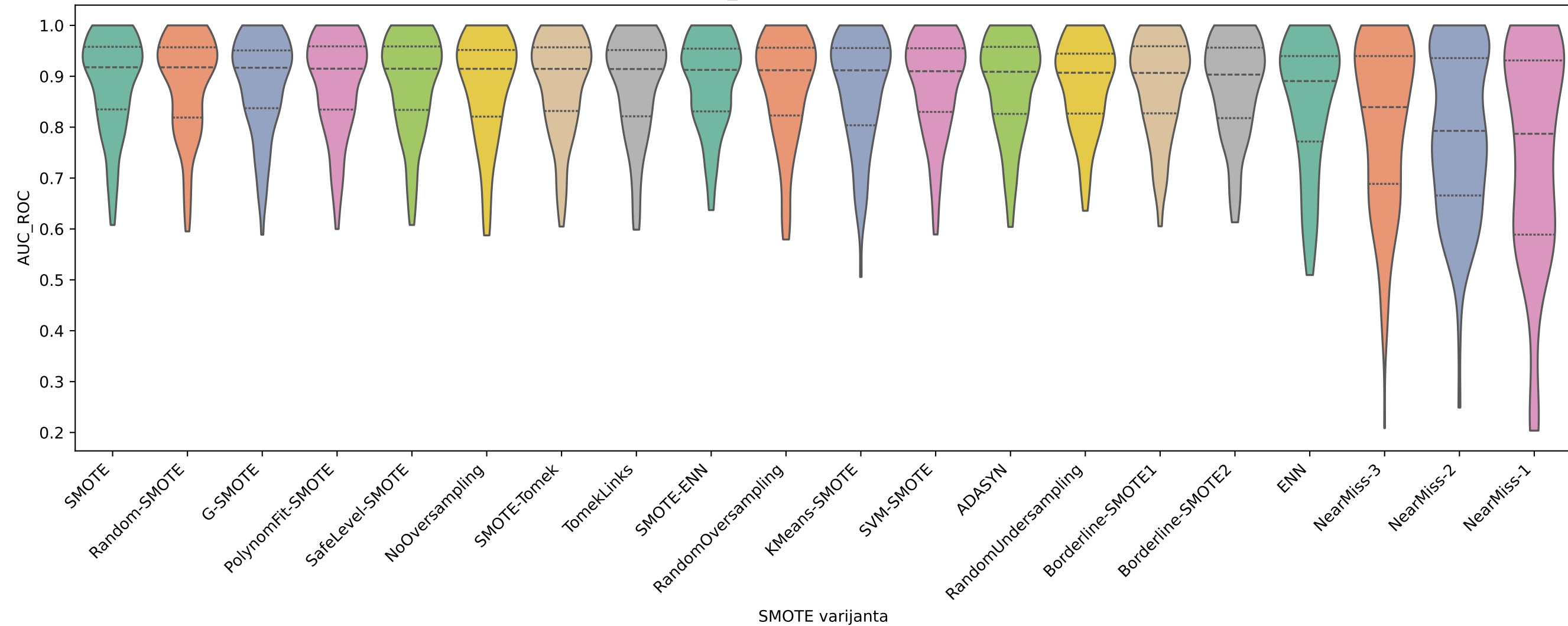
Distribucija AUC_ROC po SMOTE varijantama (violin)
