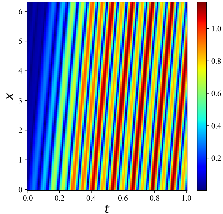
Convection (KAN) - Absolute Error
