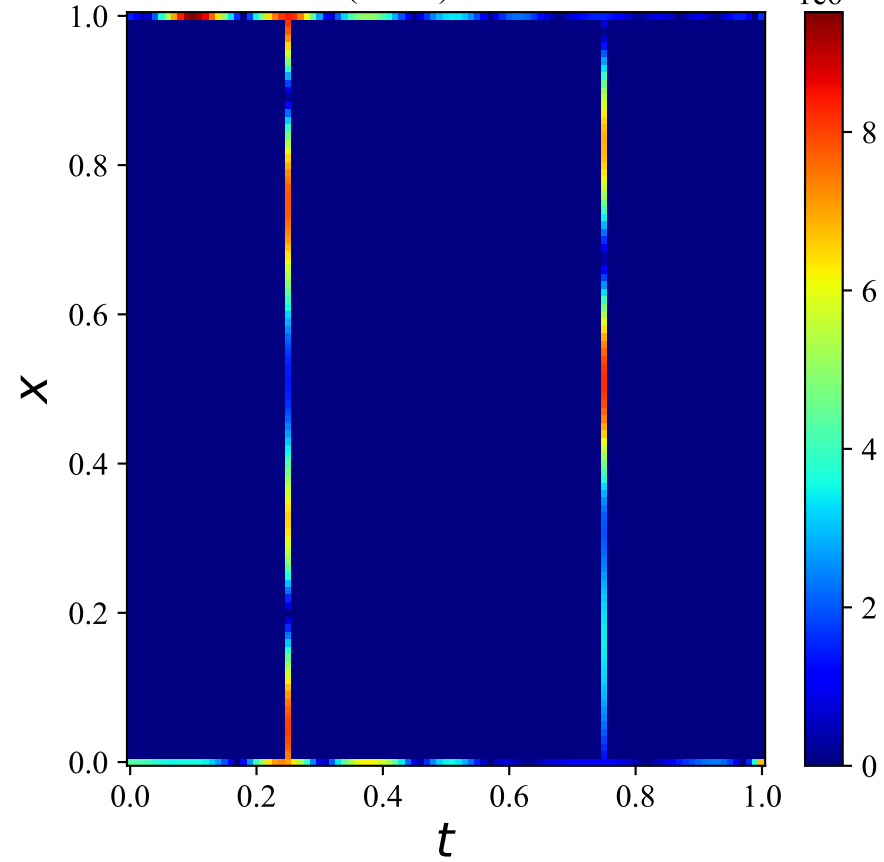
1D Wave (KAN) - Relative Error
