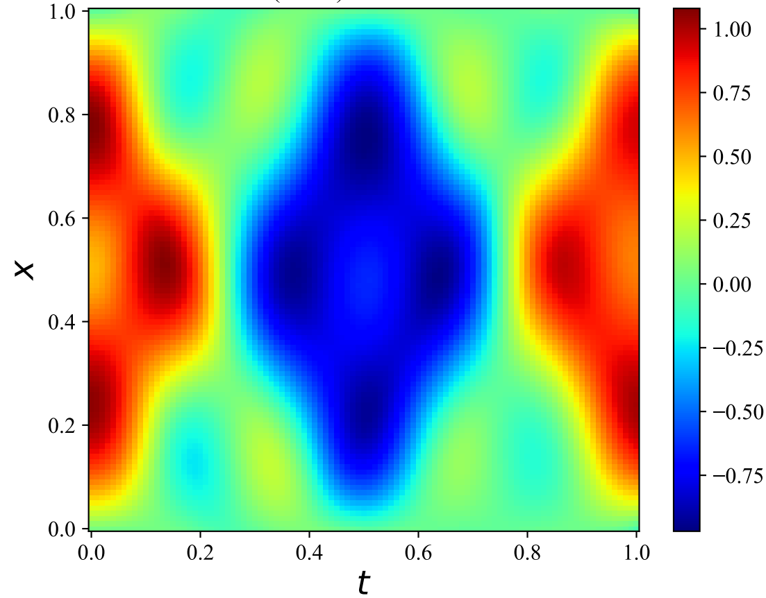
1D Wave (KAN) - Predicted Solution
