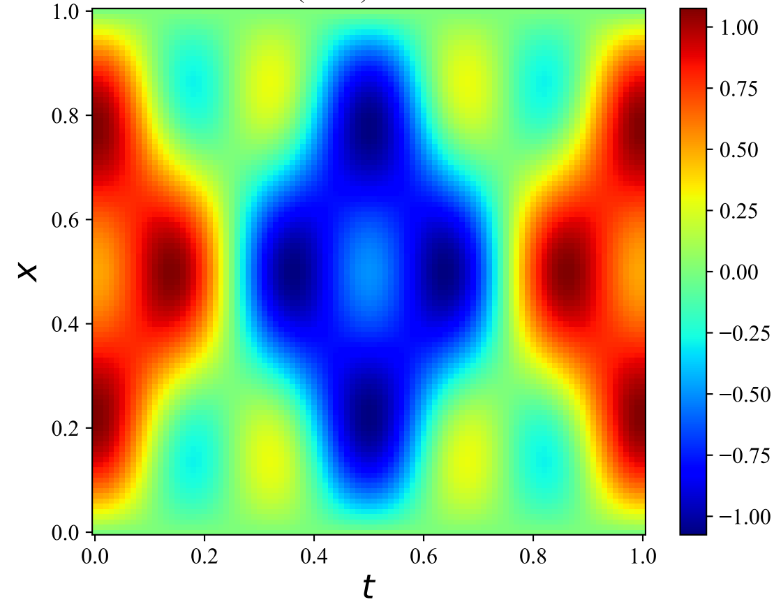
1D Wave (KAN) - Exact Solution
