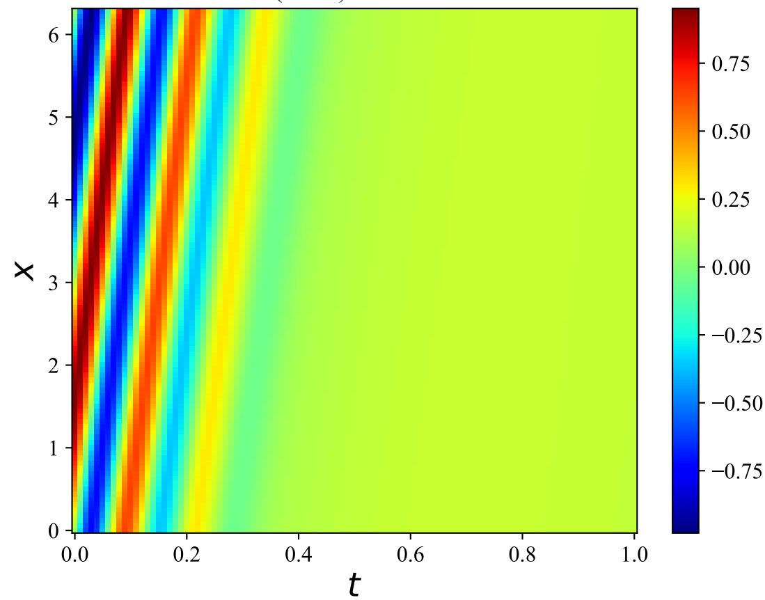
Convection (KAN) - Predicted Solution
