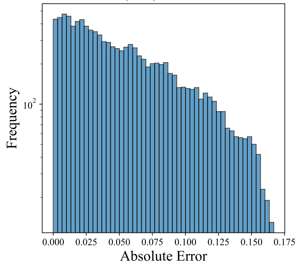
1D Wave (KAN) - Error Distribution
