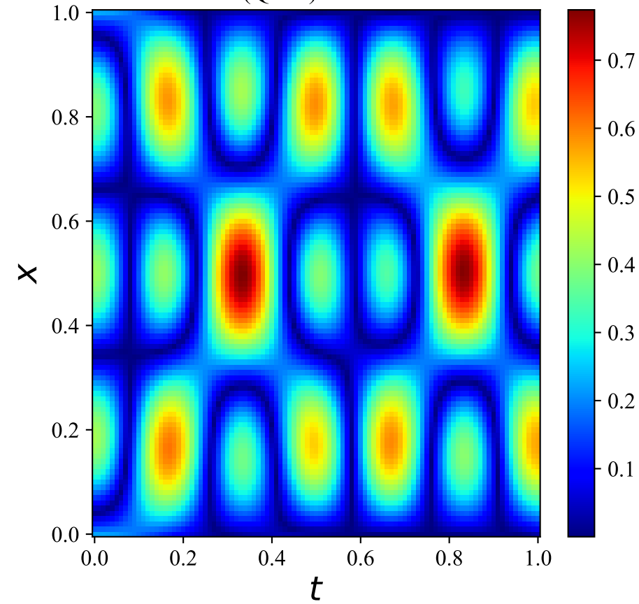
1D Wave (QRes) - Absolute Error
