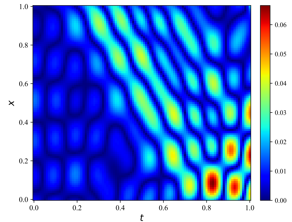
SetPINN
