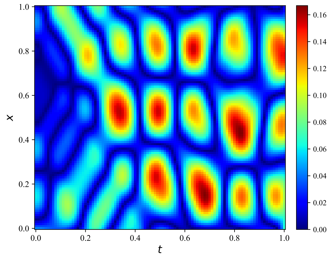
KAN
