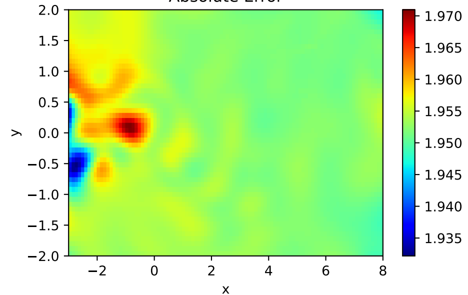
Absolute Error
