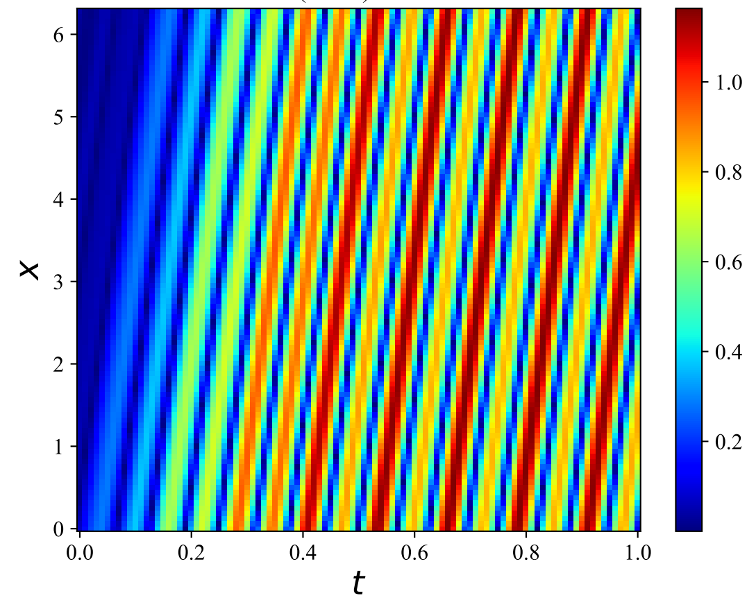
Convection (KAN) - Absolute Error
