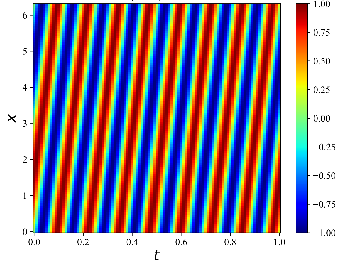
Convection (KAN) - Exact Solution
