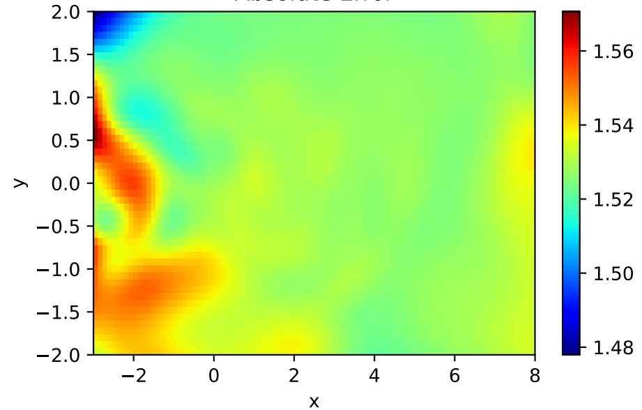
Absolute Error
