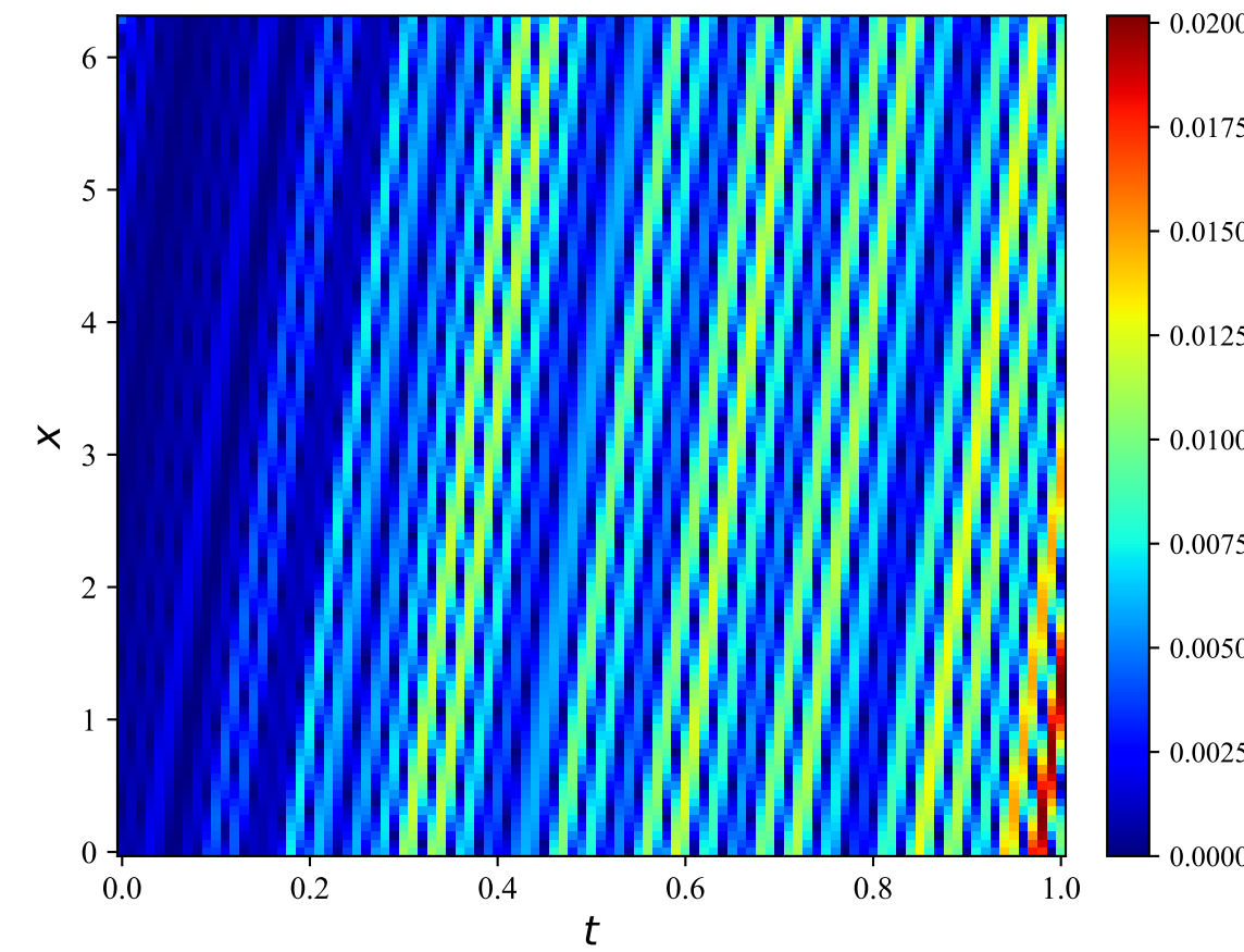
SetPINN
