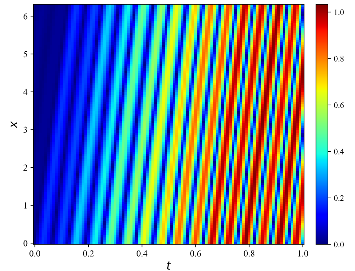
SetPINN
