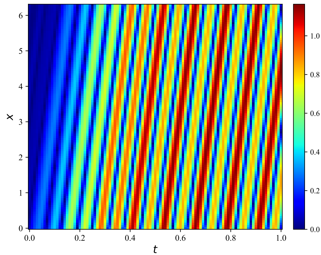
KAN
