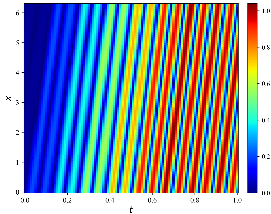
KAN
