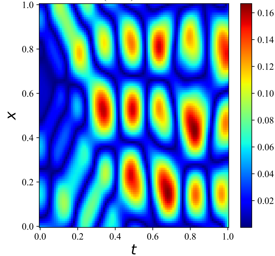
1D Wave (KAN) - Absolute Error
