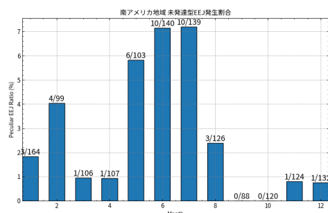
図 10 未発達型 EEJ の月ごとの発生割合 (2009-2020 年)
