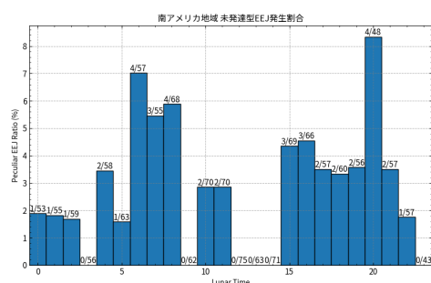
図 12 未発達型 EEJ の月齢ごとの発生割合 (2009-2020 年)
