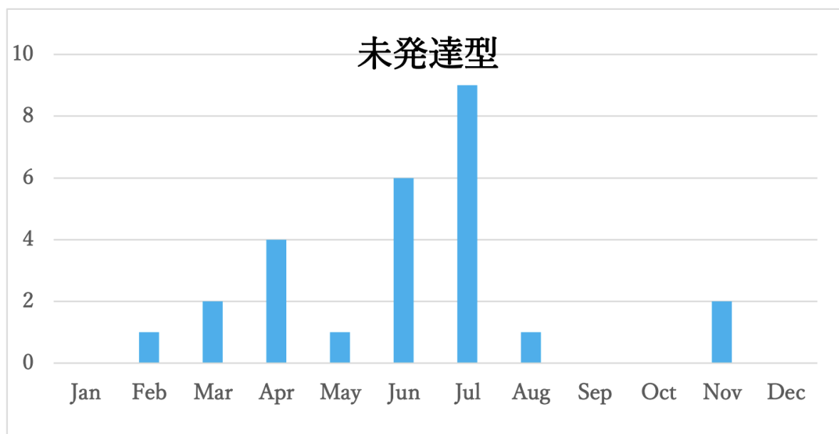
図 7 未発達型の季節変化 (池末修士論文 2024より引用)
