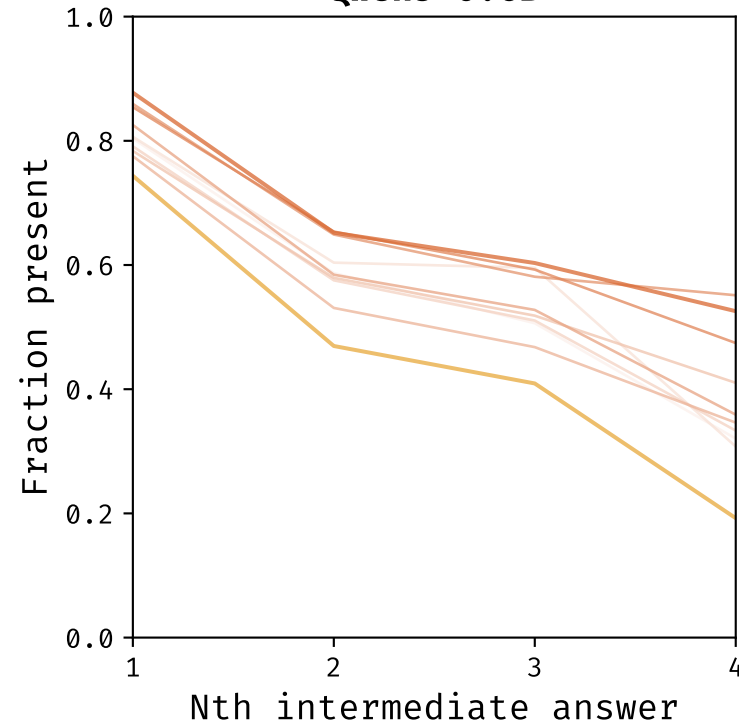
Qwen3-0.6B
