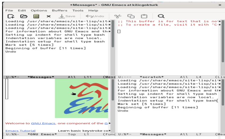
Рисунок 11: Четыре буфера
