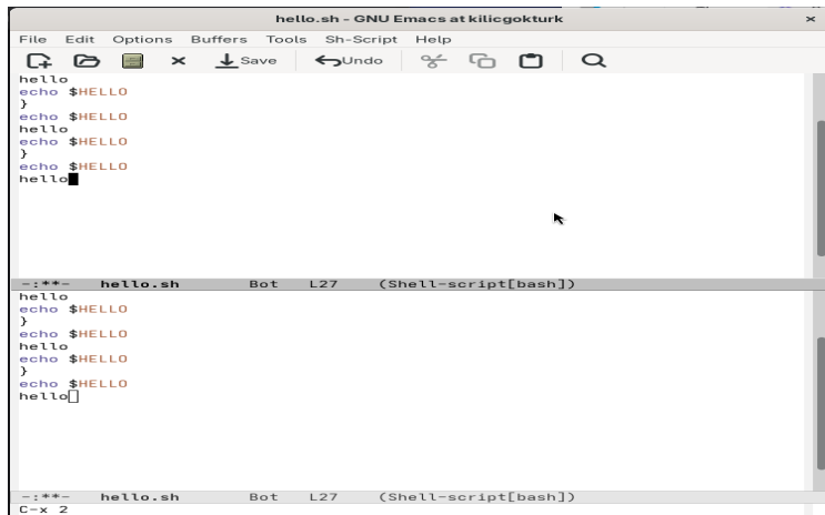
Рисунок 7: Горизонтальное разделение
