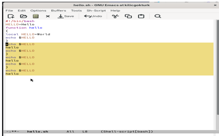
Рисунок 4: Выделение блока
