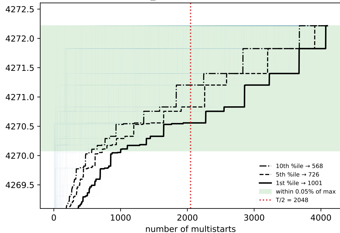
ROWP (rowp_n74) — held-out (M=4096)
