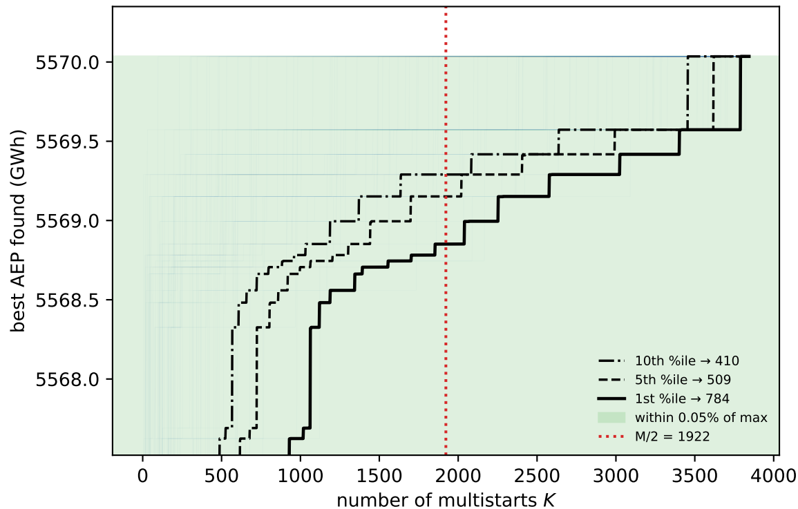
DEI (dei_n50) — training ( M = 3844 )
