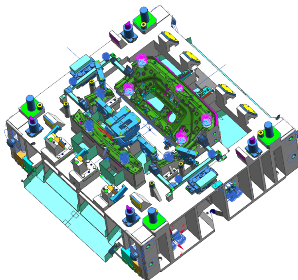
Lower die Ass' y
