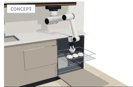
④ 식세기 인출
