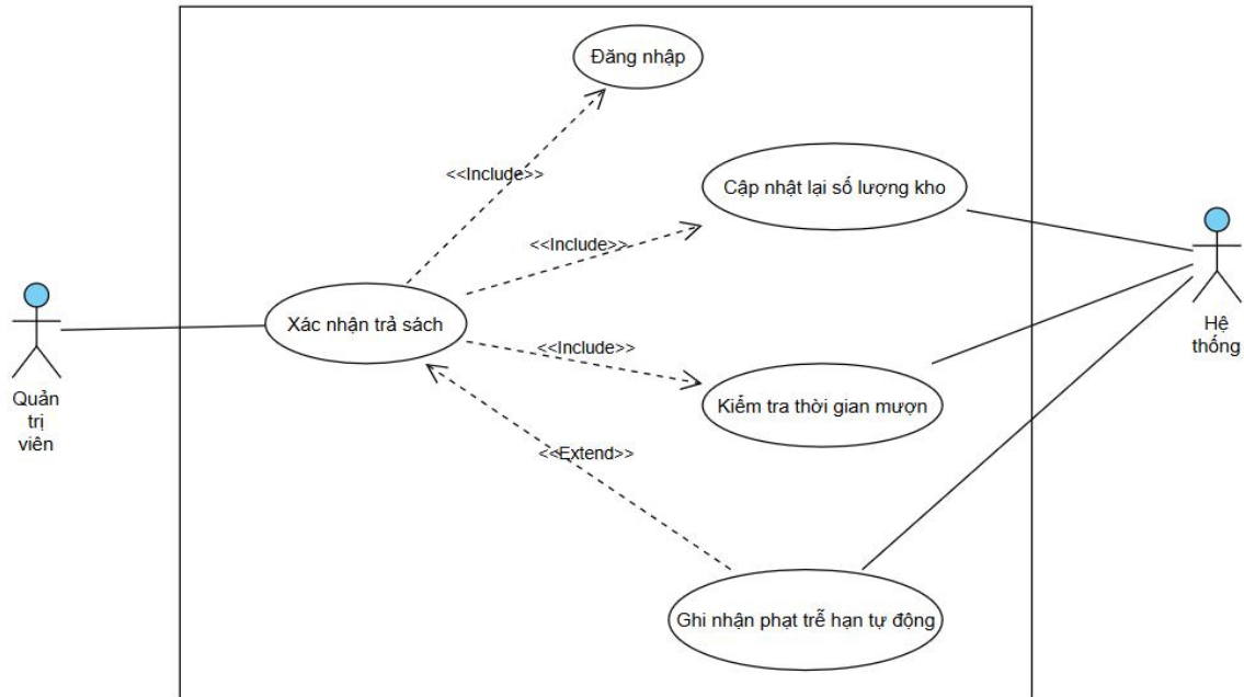
Hình 3.4 Sơ đồ Use Case xác nhận trả sách và phạt
