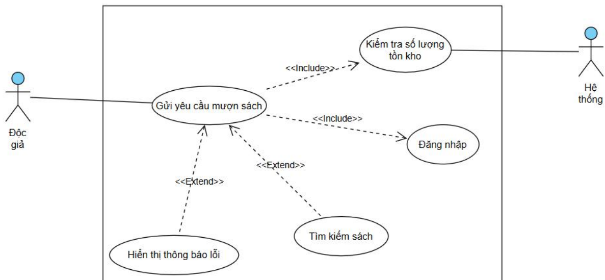
Hình 3.2 Sơ đồ Use Case gửi yêu cầu mượn sách
