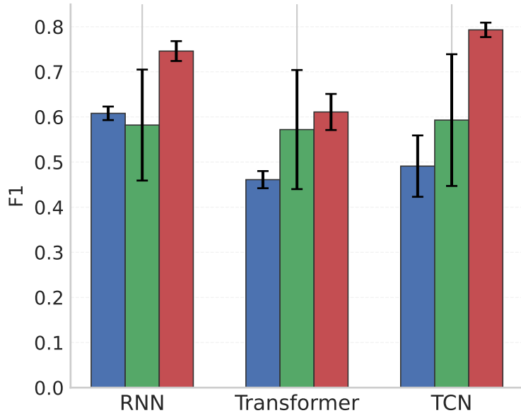
MIT-ECG
