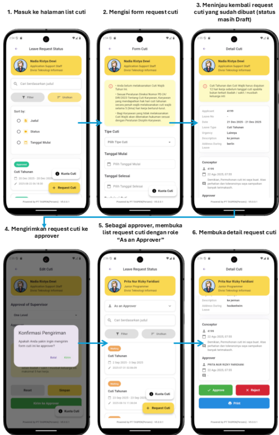
Gambar 2.3: Alur pengajuan cuti (Bagian 1)
