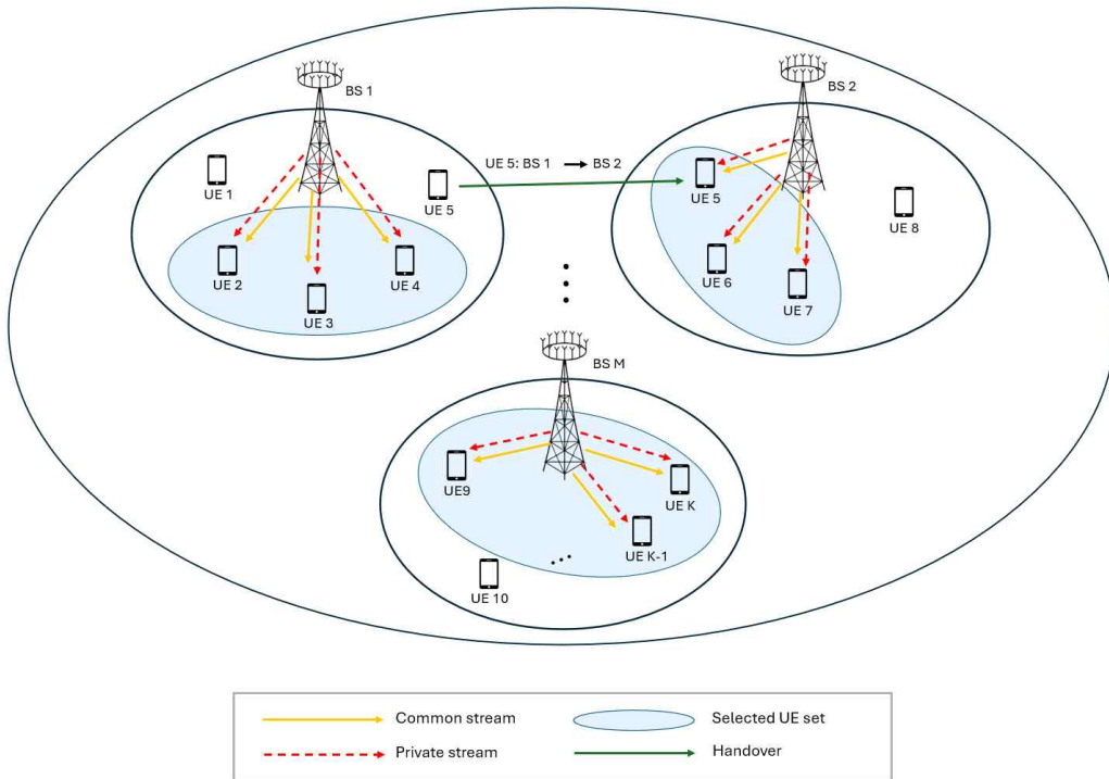
[그림 3] RSMA 기반 다중 셀 MIMO 하향링크 시스템 모델
