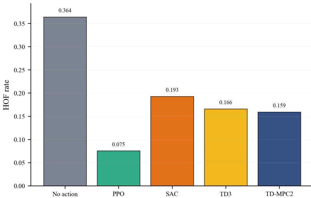
[그림 15] 이질 트래픽 환경에서의 HOF 발생률 비교
