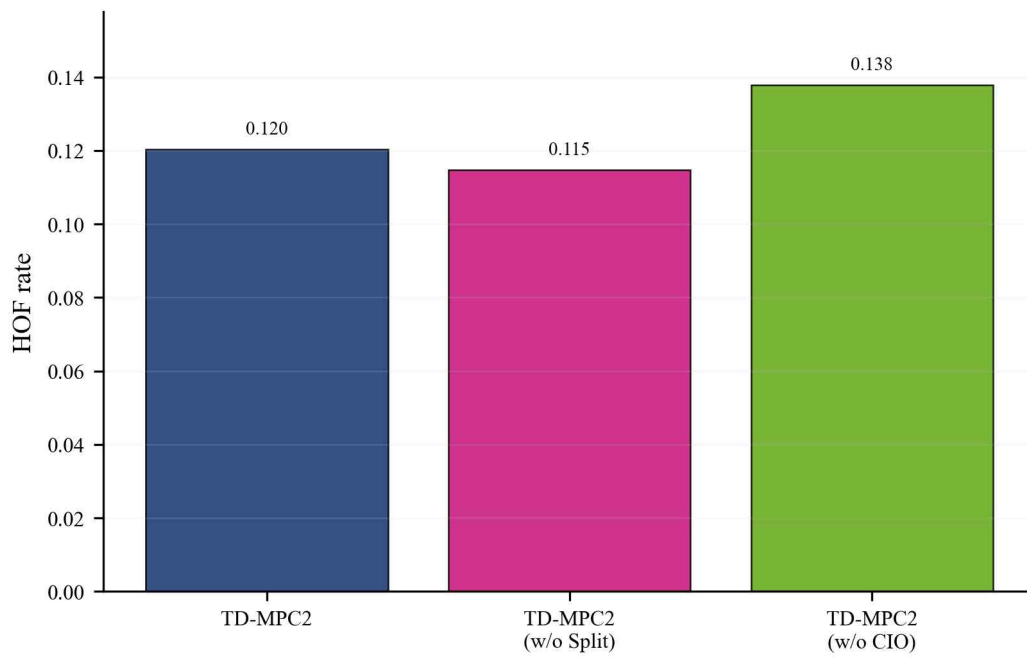
[그림 11] 개별 제어 동작에 따른 HOF 발생률 비교
