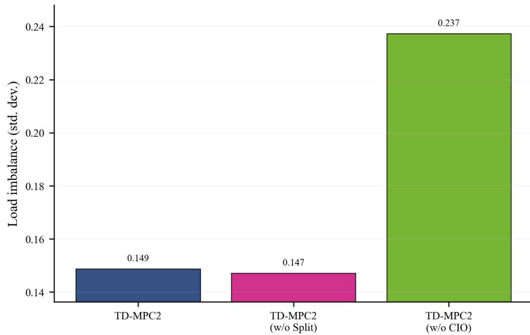
[그림 10] 개별 제어 동작에 따른 부하 불균형 비교
