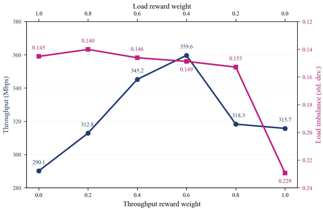
[그림 12] 보상 가중치 변화에 따른 처리량 및 부하 불균형 성능 변화
