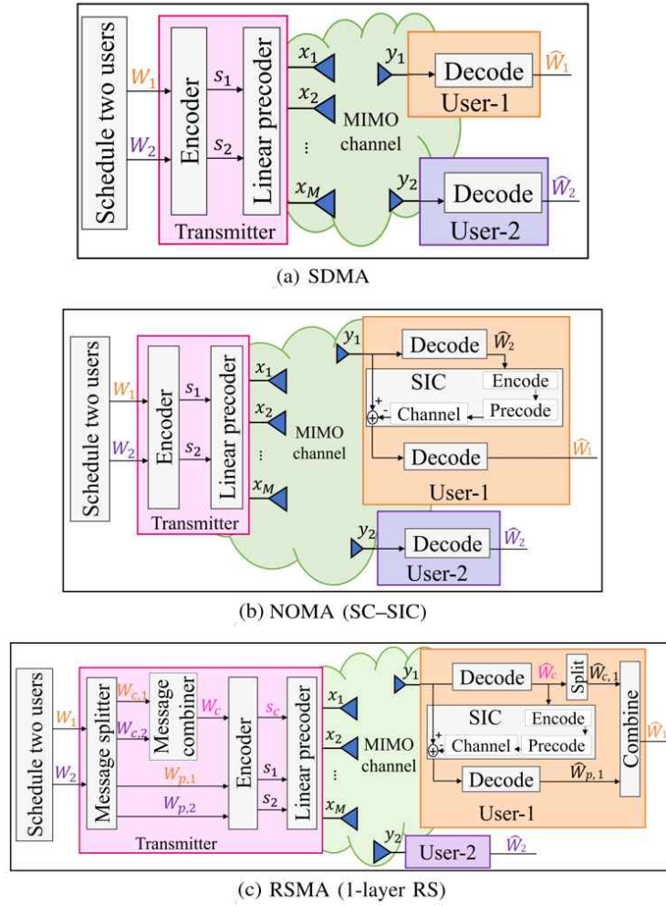
[그림 1] 하향링크 다중 안테나 시스템에서의 다중 접속 기법별 송수신 구조 비교: (a) SDMA, (b) NOMA (SC-SIC), (c) RSMA (1-layer RS) [3]
