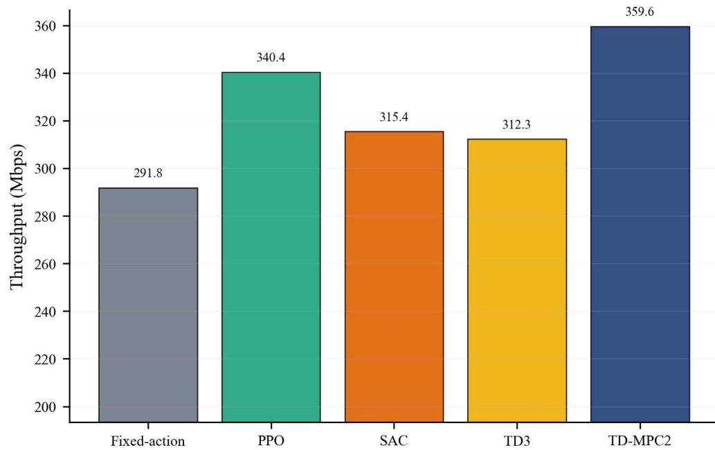
[그림 6] 시스템 처리량 비교
