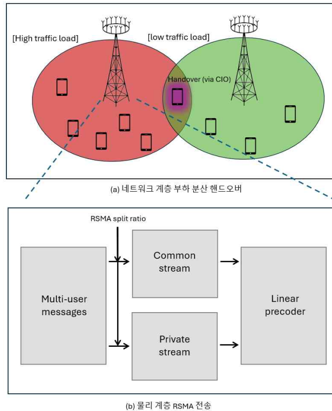
[그림 2] 트래픽 부하 불균형 해소 및 처리량 향상을 위한 교차 계층 공동 제어 개요: (a) 네트워크 계층 부하 분산 핸드오버, (b) 물리 계층 RSMA 전송
