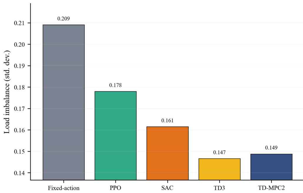
[그림 7] 셀 간 부하 불균형 비교
