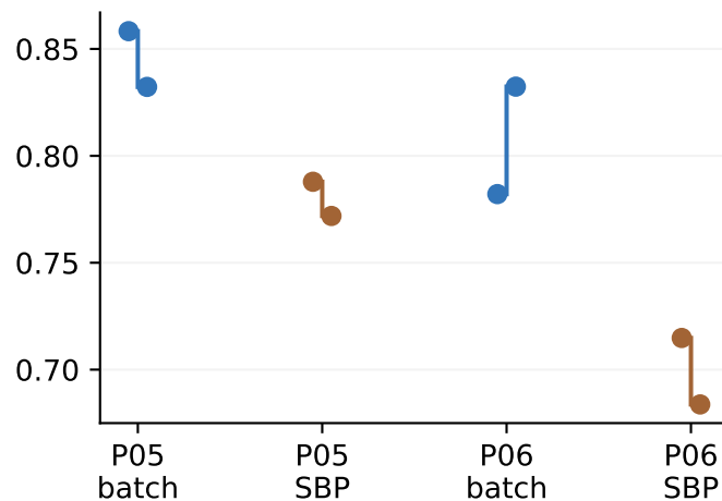
skin ssim
