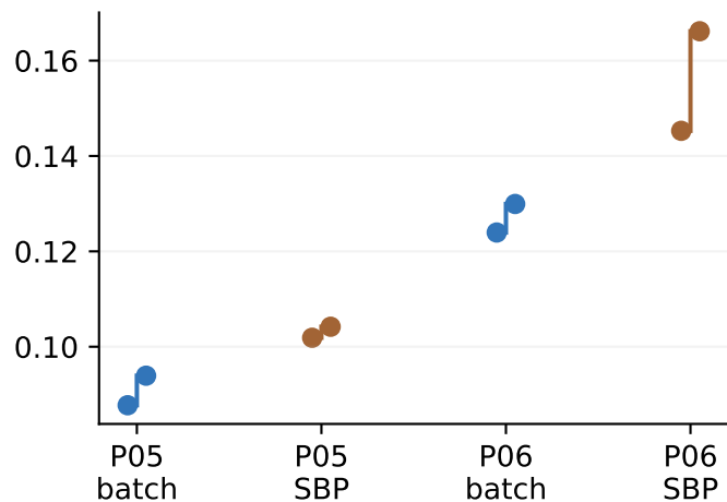
skin mae
