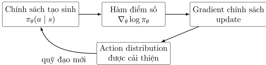
Hình 4: Sơ đồ cho thấy vai trò của hàm điểm số: cùng đại lượng \nabla_{\theta} \log \pi_{\theta} xuất hiện trong gradient chính sách và trong generative model, nên chính sách tạo sinh có thể được cập nhật bằng tín hiệu RL.
