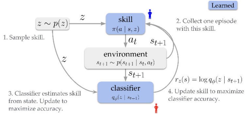
Hình 15: Minh họa Skill Learning (DIAYN): agent học các skill đa dạng (chạy, nhảy, cân bằng) bằng cách tối đa hóa thông tin tương hỗ giữa skill label z và quỹ đạo \tau . Discriminator q(z|s) học nhận biết skill từ trạng thái, tạo ra intrinsic reward cho chính sách. Nguồn: [7].
