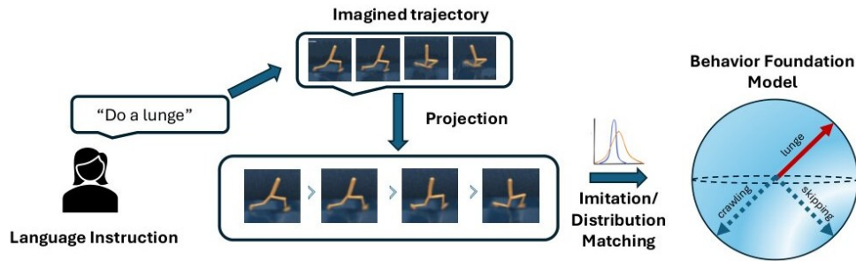
Hình 13: Framework của RLZero gồm 3 bước: Imagine (tưởng tượng video từ ngôn ngữ), Project (chiếu về không gian quan sát của agent), Imitate (suy ra chính sách zero-shot). Nguồn: [19].
