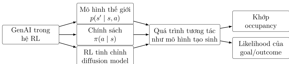
Hình 10: Tổng hợp hai mức phân tích của tutorial. Phần I đặt generative models vào hệ RL. Phần II xem quá trình tương tác của agent như một mô hình tạo sinh tạo ra occupancy, goal và outcome distribution.
