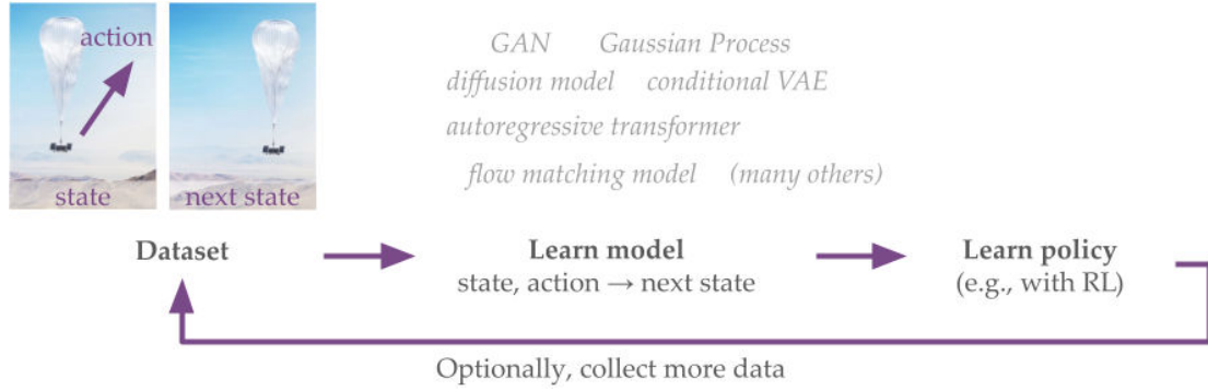
Hình 2: Pipeline model-based RL với mô hình thế giới: generative model được huấn luyện để học dynamics từ transition data, sau đó hỗ trợ học chính sách. Nguồn hình: Figure 3 trong [7].
