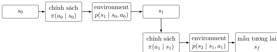
Hình 8: Quá trình tương tác tạo sinh: mỗi bước chính sách sinh action, environment sinh state kế tiếp, và toàn bộ vòng lặp tạo ra mẫu tương lai s_f .
