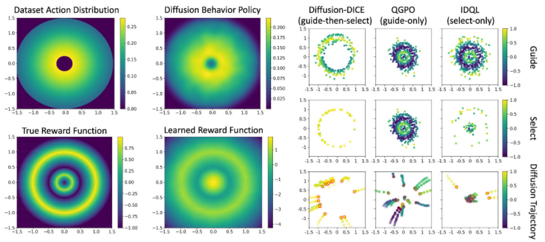
Hình 6: Toycaze 2D bandit của Diffusion-DICE: action trong bộ dữ liệu nằm trong vùng hình khuyên; true reward cao ở outer circle; learned reward overestimate inner circle; Diffusion-DICE giảm khai thác lỗi tốt hơn các hướng guide-only hoặc select-only. Nguồn hình: Figure 7 trong [7].
