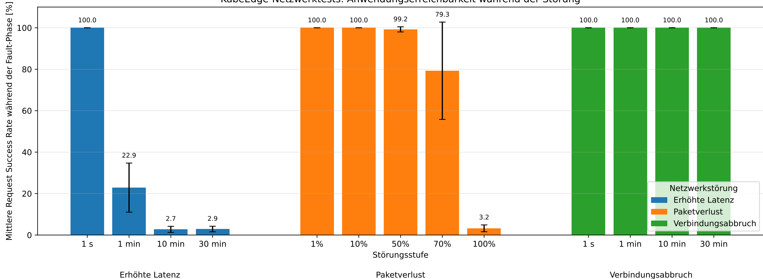
KubeEdge-Netzwerktests: Anwendungserreichbarkeit während der Störung
