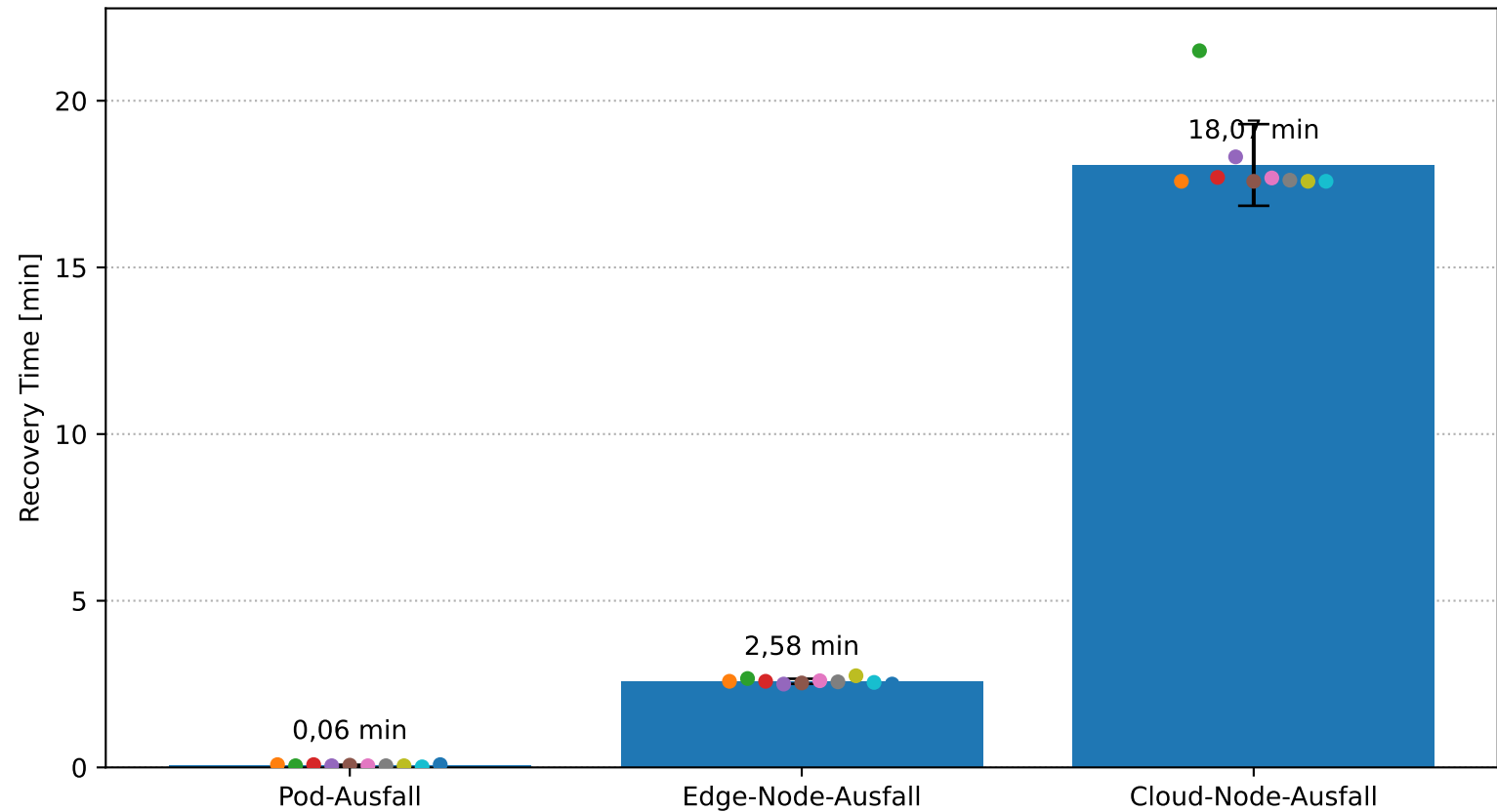
KubeEdge: Recovery Time bei Pod- und Node-Ausfällen
