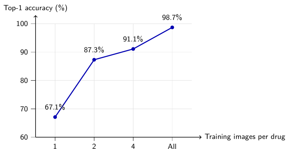
図 3 1 薬剤あたりの学習元画像枚数と Top-1 正答率 (33 薬剤)
