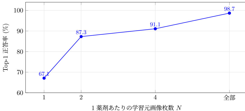
図3 1 薬剤あたりの学習元画像枚数と Top-1 正答率 (33 薬剤. 横軸の「全部」は 5~8 枚)
