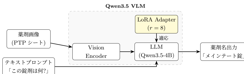
図 1 提案手法の処理フロー：薬剤画像とテキストプロンプトを Qwen3.5 に入力し、LoRA アダプタで薬剤画像データに適応させて薬剤名を出力する
