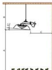
Detalle de suspensión del radiador
