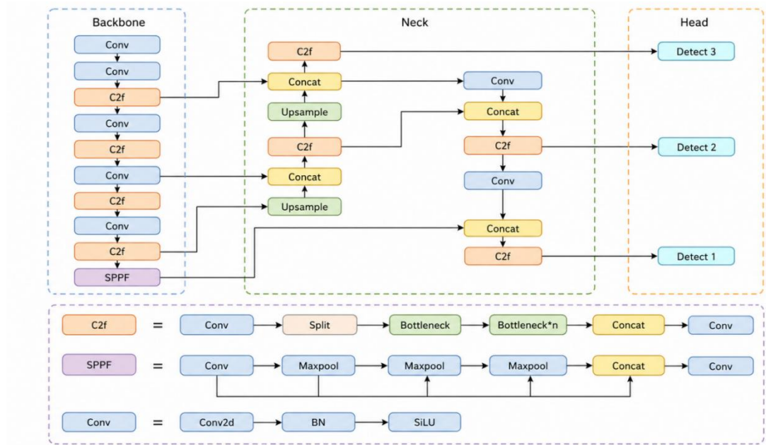
图 2-2 YOLOv8 网络结构图
