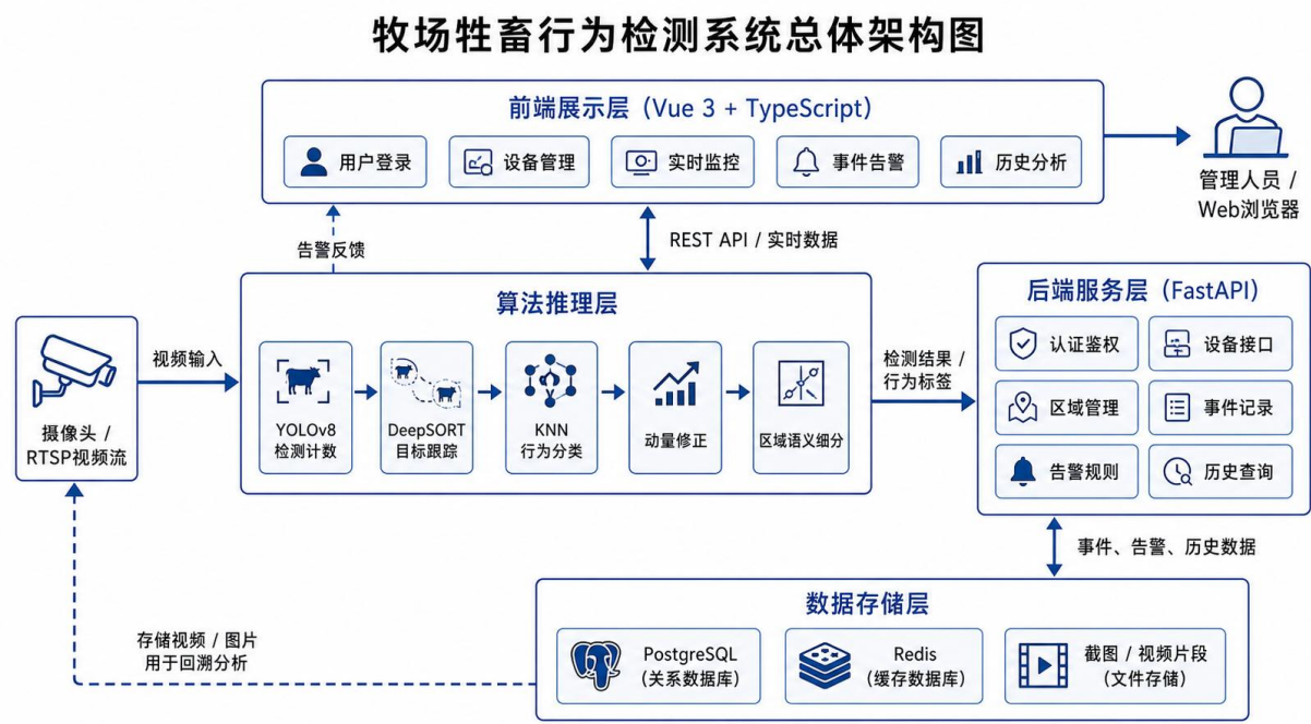
图 5-1：系统总体架构图
