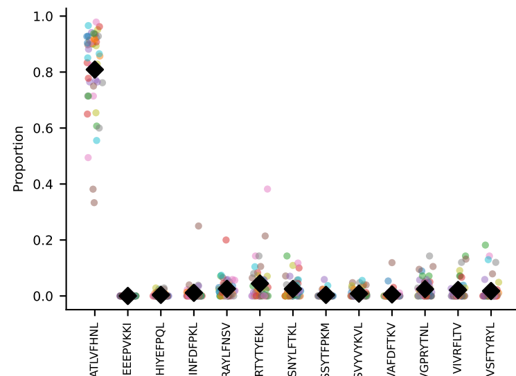
#124 AV13-1-CALEQGGSAKLIF-AJ57_BV12-2-CASSLEGADTEVFF-BJ1-1 coh=0.963, n=48
