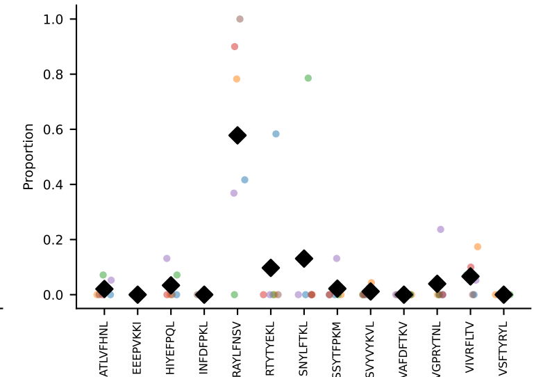
#20 AV7-2-CAATGNTGKLIF-AJ37_BV19-CASSIRIAEQFF-BJ2-1 coh=0.465, n=8
