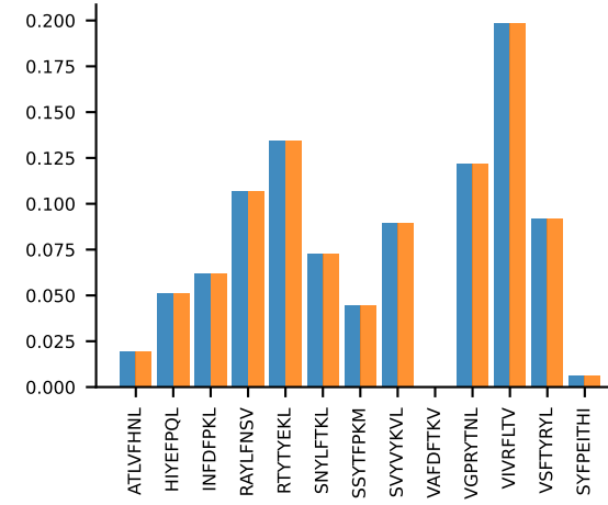
AV5-1-CSASTGGFASALTf-AJ35_BV2-CASSQDGAGANSDYTF-BJ1-1AV5-1-CSASTGGFASALTf-AJ35_BV2-CASSQDGAGANSDYTF-BJ1-1 PROP n:6→6
