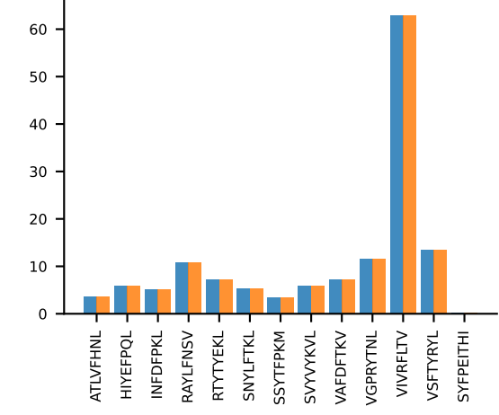
AV5-1-CSASTGGFASALTf-AJ35_BV2-CASSQDGAGANSDYTF-BJ1-1AV5-1-CSASTGGFASALTf-AJ35_BV2-CASSQDGAGANSDYTF-BJ1-1 MEAN n:6→6
