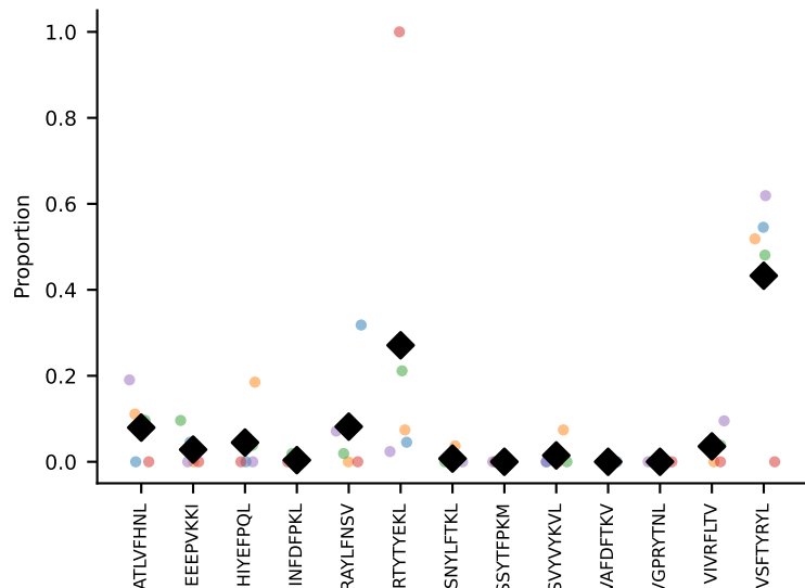
#5 AV10N-CAASMDTGGLSGKLTf-AJ2_BV16-CASSLNWGANYAEQFF-BJ2-#6 AV16/DV11-CAMREGGGYKVVf-AJ12_BV13-2-CASGARTYNIAEQFF-BJ2-1 coh=0.386, n=13
