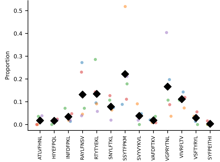
#120 AV5-1-CSASISGGNYKPT F-AJ6_BV29-CASSLRKTDTQYF-BJ2-5 coh=0.645, n=5
