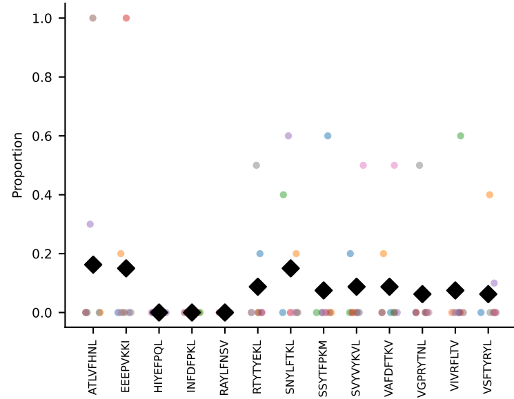
#102 AV10N-CAASMAGGNYKPTF-AJ6_BV1-CTCSADSGGNYAEQFF-BJ2-1 coh=0.095, n=8
