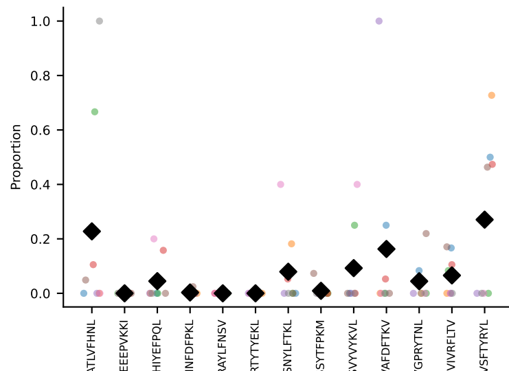
#47 AV6-6-CALGDTGGYKVV-F-AJ12_BV14-CASSFWNYAEQFF-BJ2-1 coh=0.268, n=11
