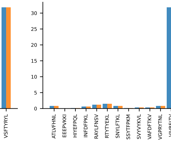
AV6-3-CALGDHMGYKLTf-AJ9_BV26-CASSLGGYAEQFF-BJ2-1 MEAN n:6→6
