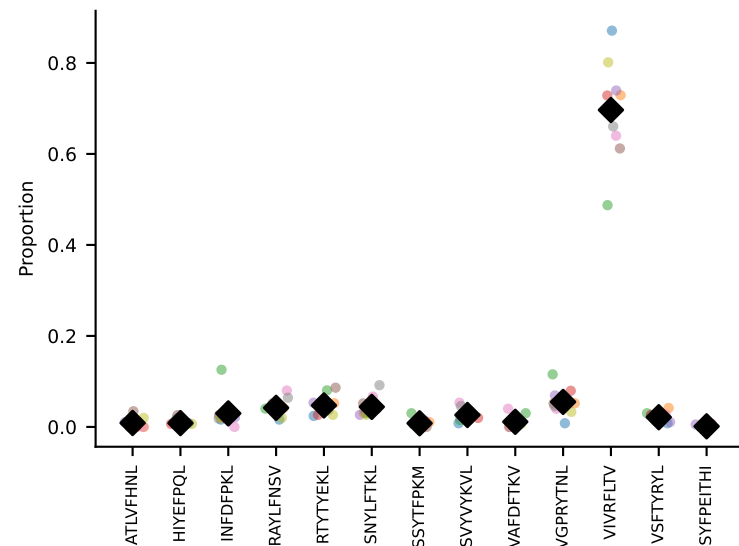
#33 AV2-CIVTDSYSNNRTL-AJ7_BV1-CTCSAGRGDAAEQFF-BJ2-1 coh=0.975, n=35
