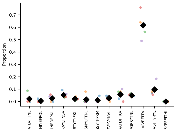
#33 AV14-3-CAASPNAVIVf-AJ30_BV16-CASSFSGTGEYEQYF-BJ2-7 coh=0.969, n=5
